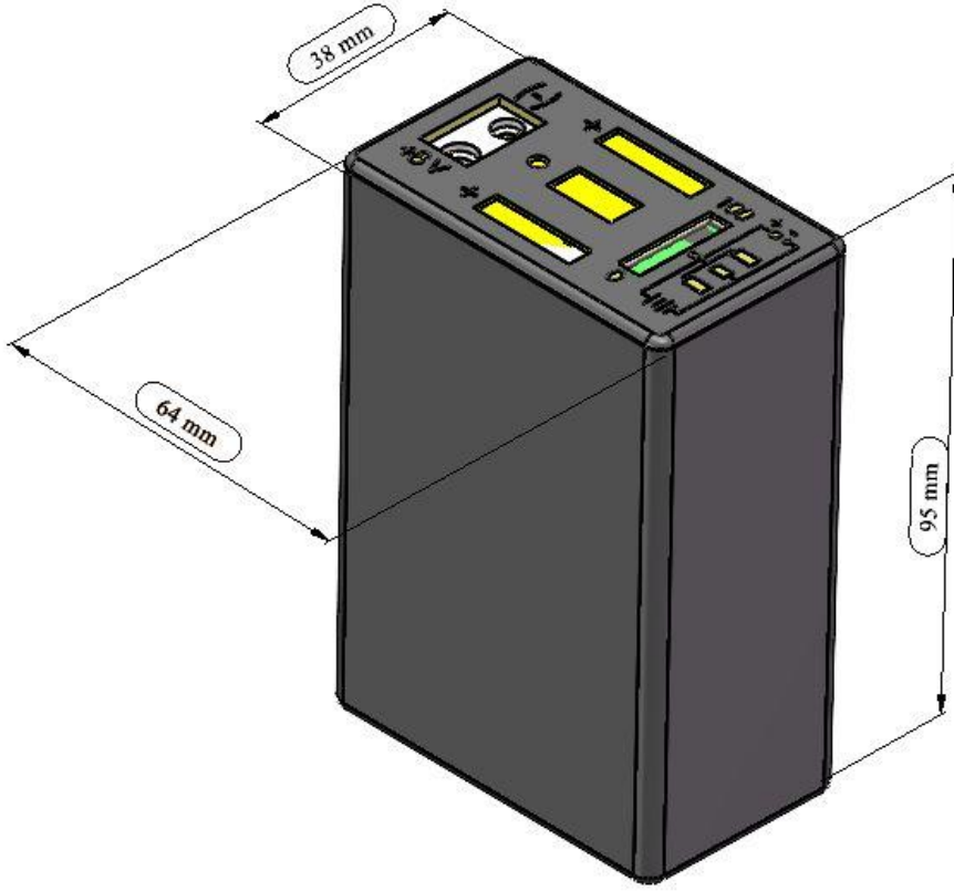
Şekil 3. Batarya Ölçüleri(mm)
