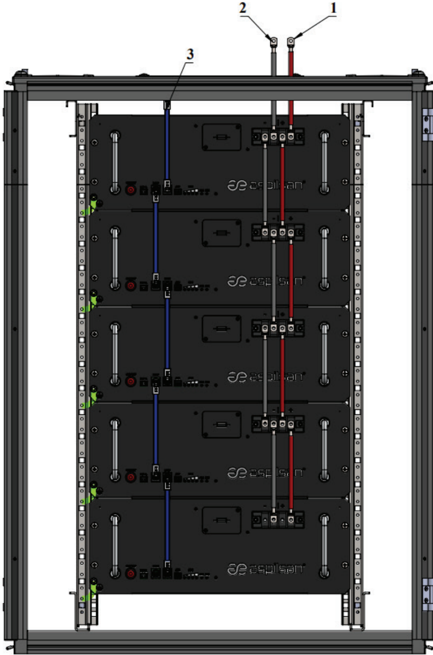
Şekil 7: Paralel Bağlama Şeması
