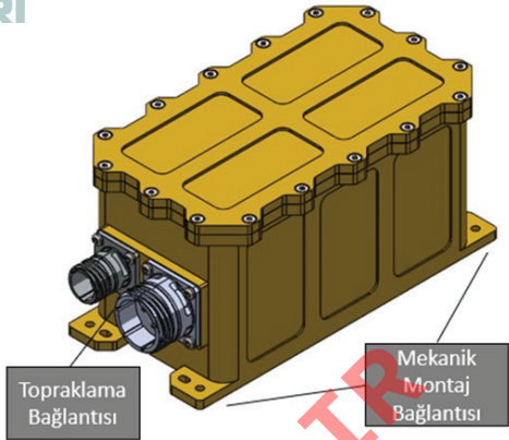
Şekil 1. Batarya Görünümü
