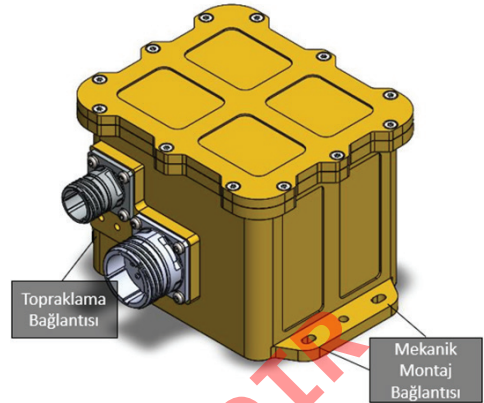
Şekil 1. Batarya Görünümü
